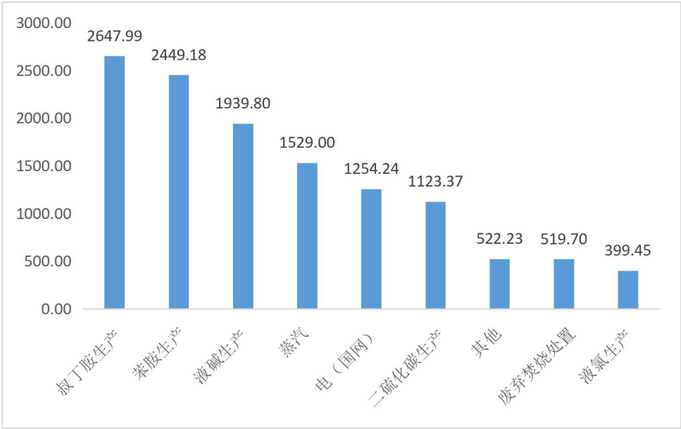
图 4 硫化促进剂 NS (TBBS) 过程贡献分析
