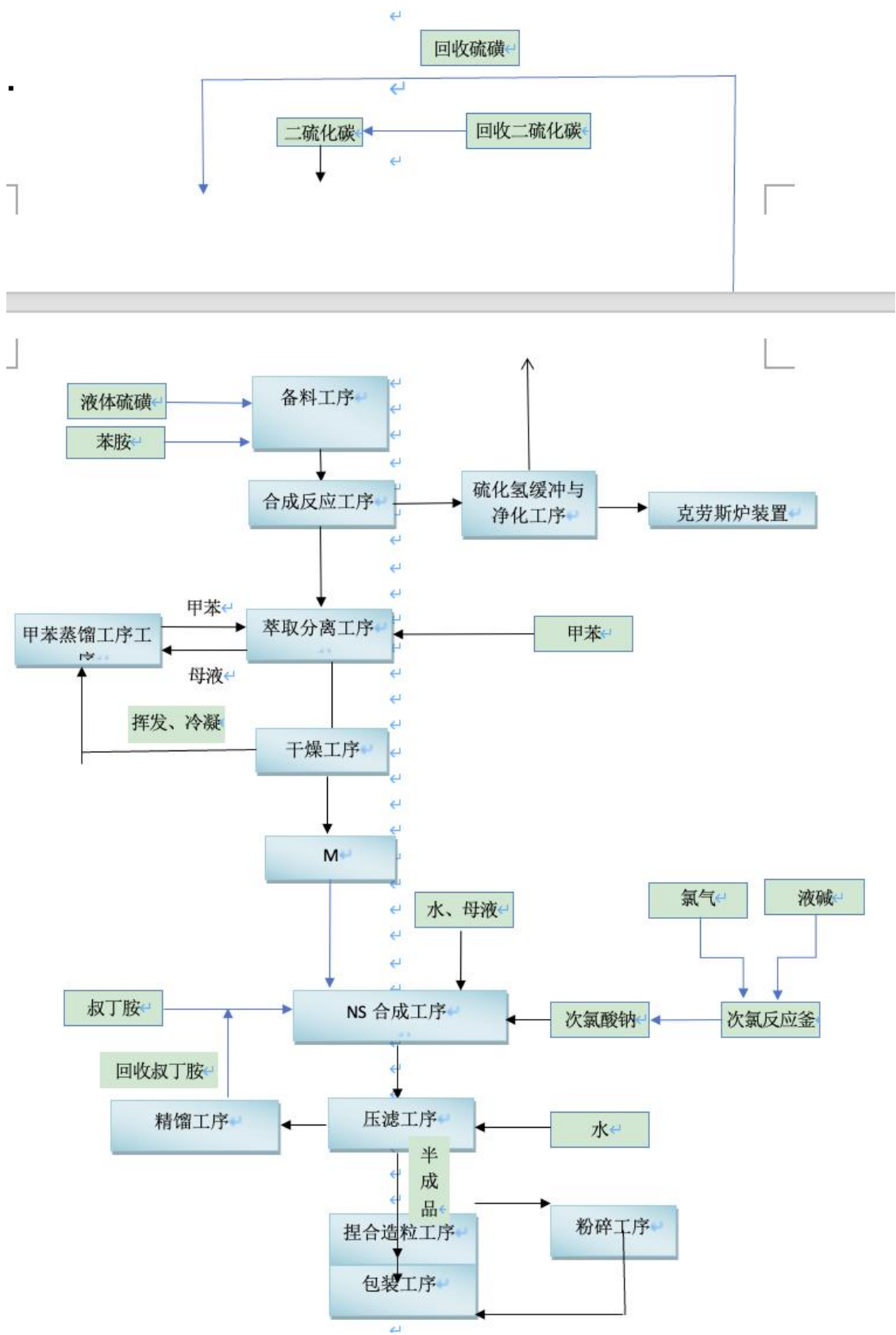
图 2 产品生产工艺流程图
